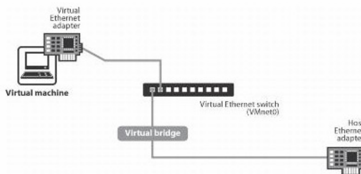
Hình 4: Cấu trúc mạng Bridged Networking
