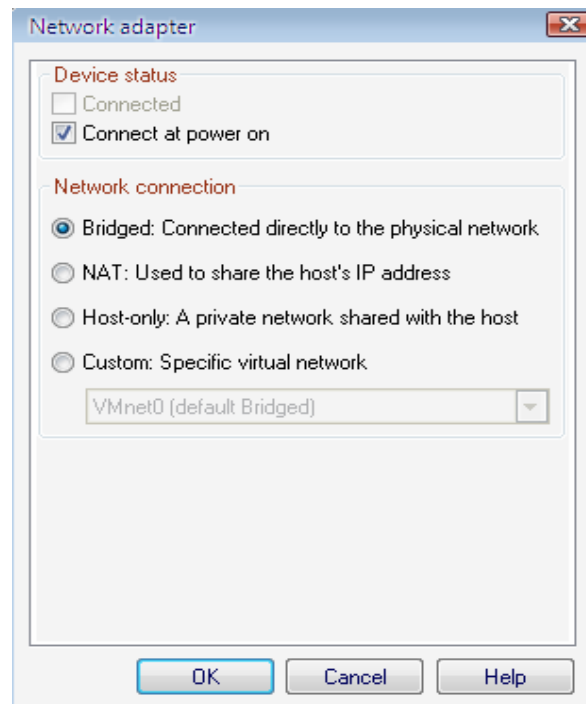
Hình 3: Chọn lựa cấu hình mạng
