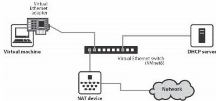
Hình 5: Cấu trúc mạng NAT
