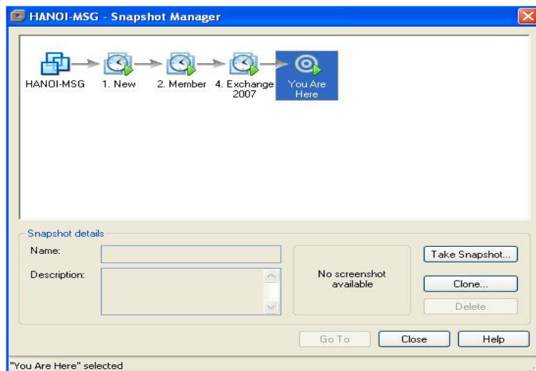
Hình 17: Tạo snapshot
